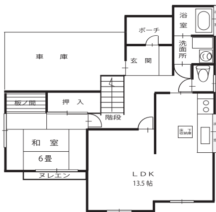
1階
